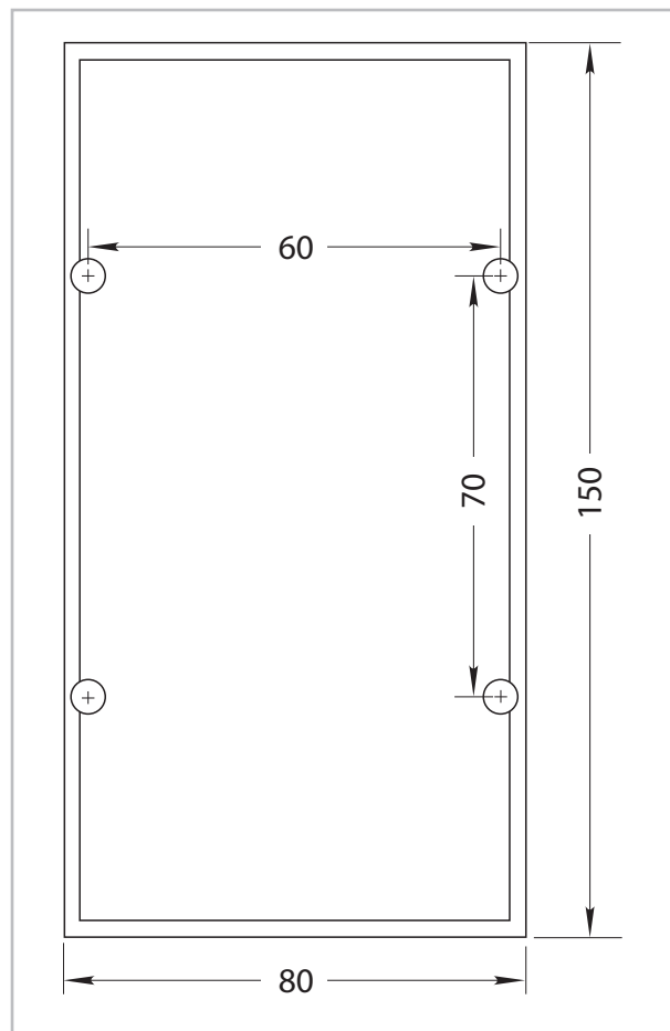
Abb. 61: Aufbau und Maße des Wandhalters (Alle Angaben in mm)
