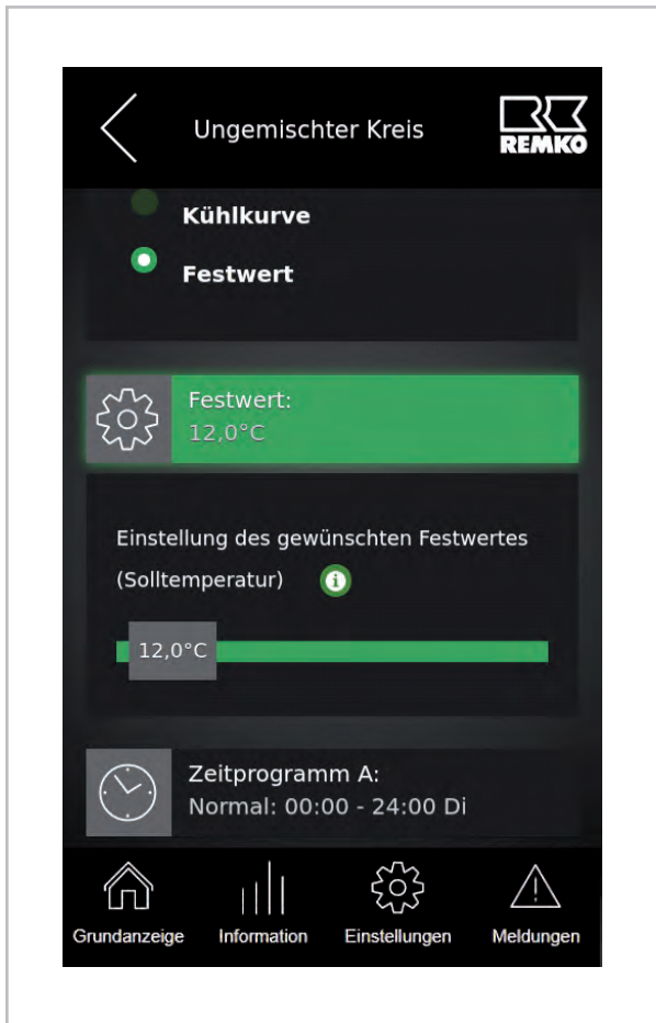
Abb. 41: Einstellen des Festwertes (Solltemperatur)
