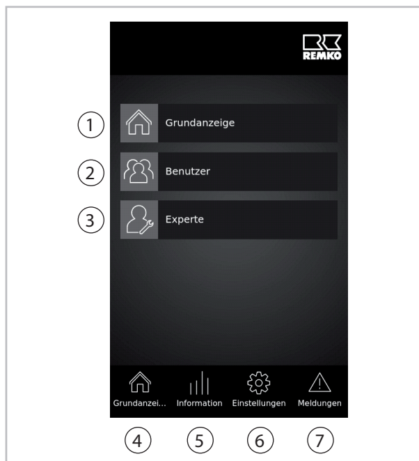
Abb. 1: Bedienelemente des Smart-Control Touch
