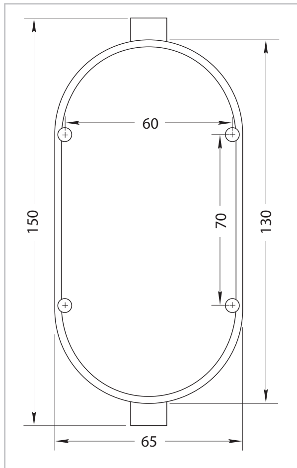
Abb. 63: Aufbau und Maße des Wandhalters (Alle Angaben in mm)
