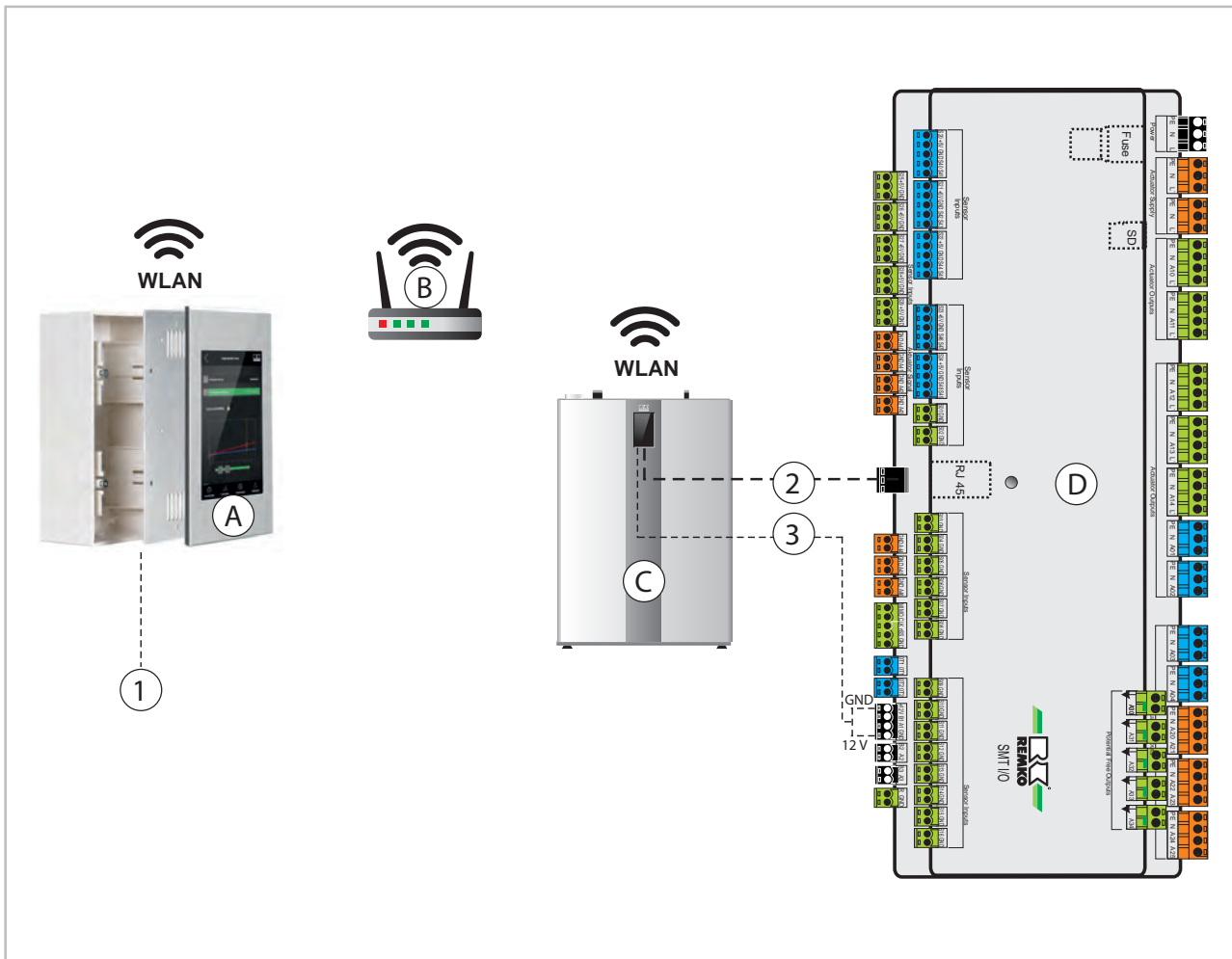
Abb. 64: Anschluss an das I/O-Modul
